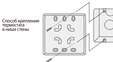
Кронштейн NR-15
